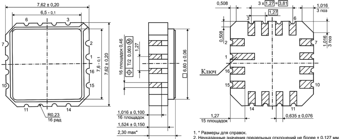
Рис. 4. Корпус 5119.16-A Размеры в миллиметрах.
